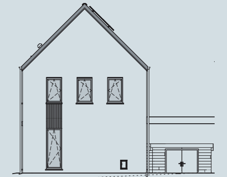
Façade avant
